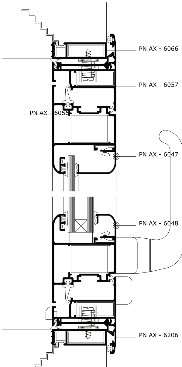
DETALLE BORDE CURVO
