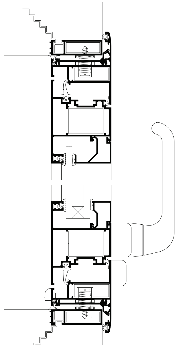
DETALLE BORDE RECTO
