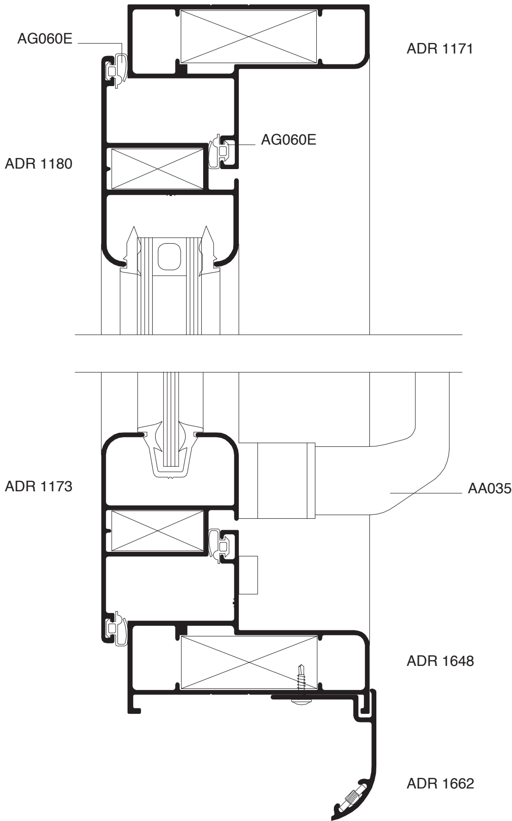
Secciones (Escala 1:1)
