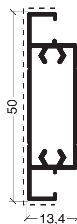
ADR 11 Trav. mosquitero 0,473 kg/m
