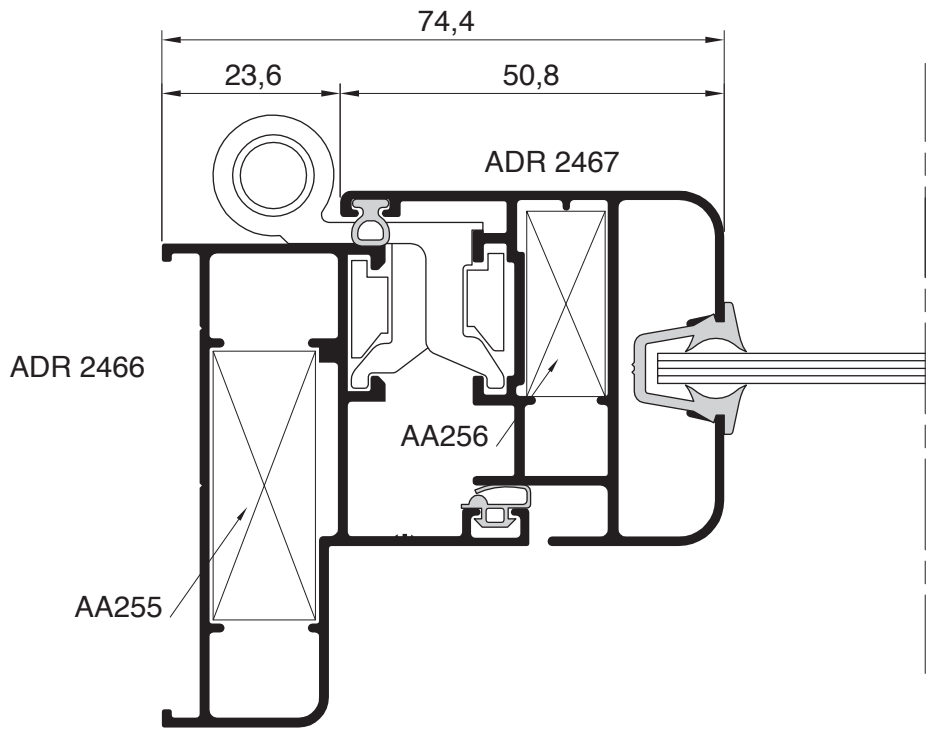
Secciones (Escala 1:1)
