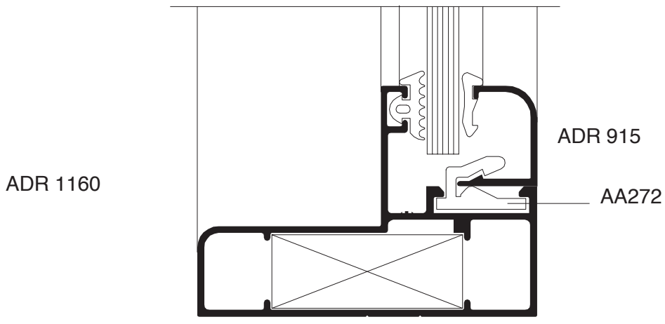
Secciones (Escala 1:1)
