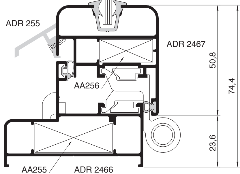
Secciones (Escala 1:1)
