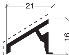
ADR 255 Vierteaguas 0,201 kg/m
