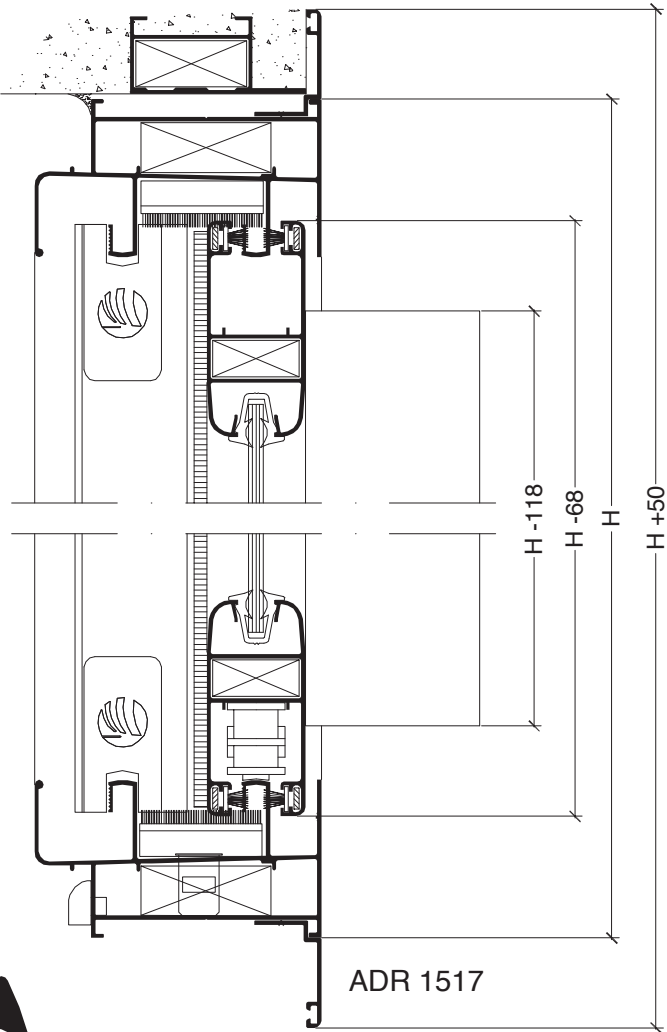
Ventana corrediza 2 hojas corte a 45° con refuerzos centrales
