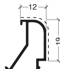
ADR 914 Contravidrio curvo 12 mm 0,209 kg/m
