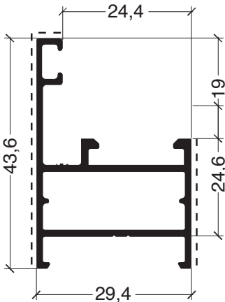
Escuadra AA256
