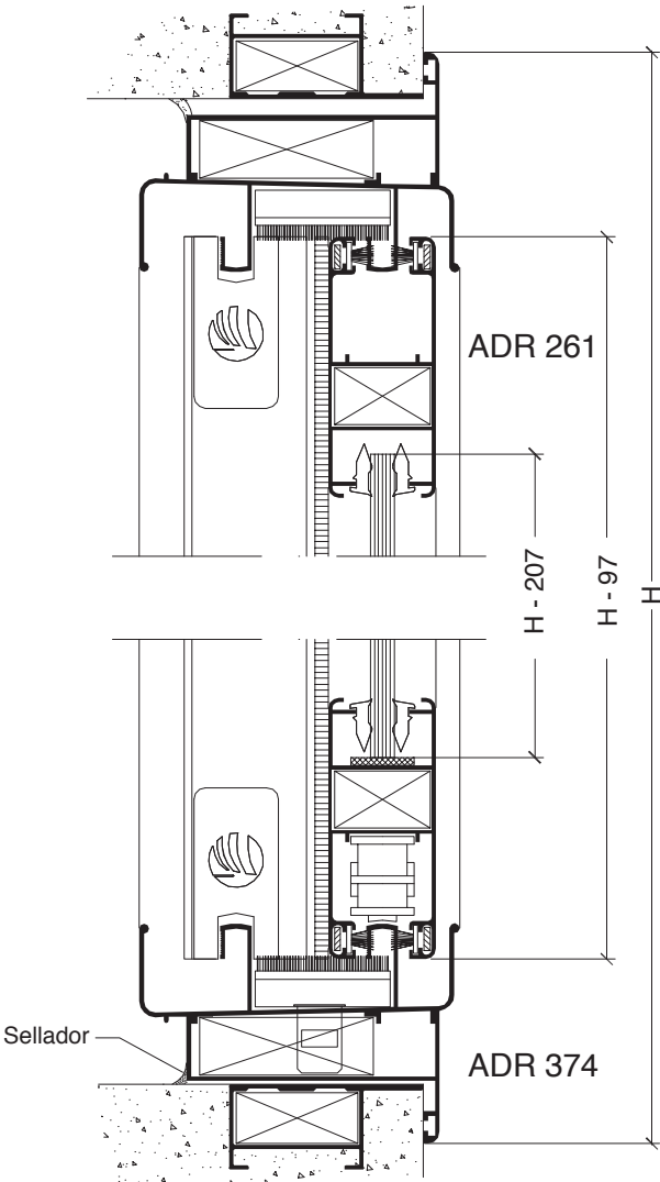
Ventana corrediza 2 hojas corte a 45°
