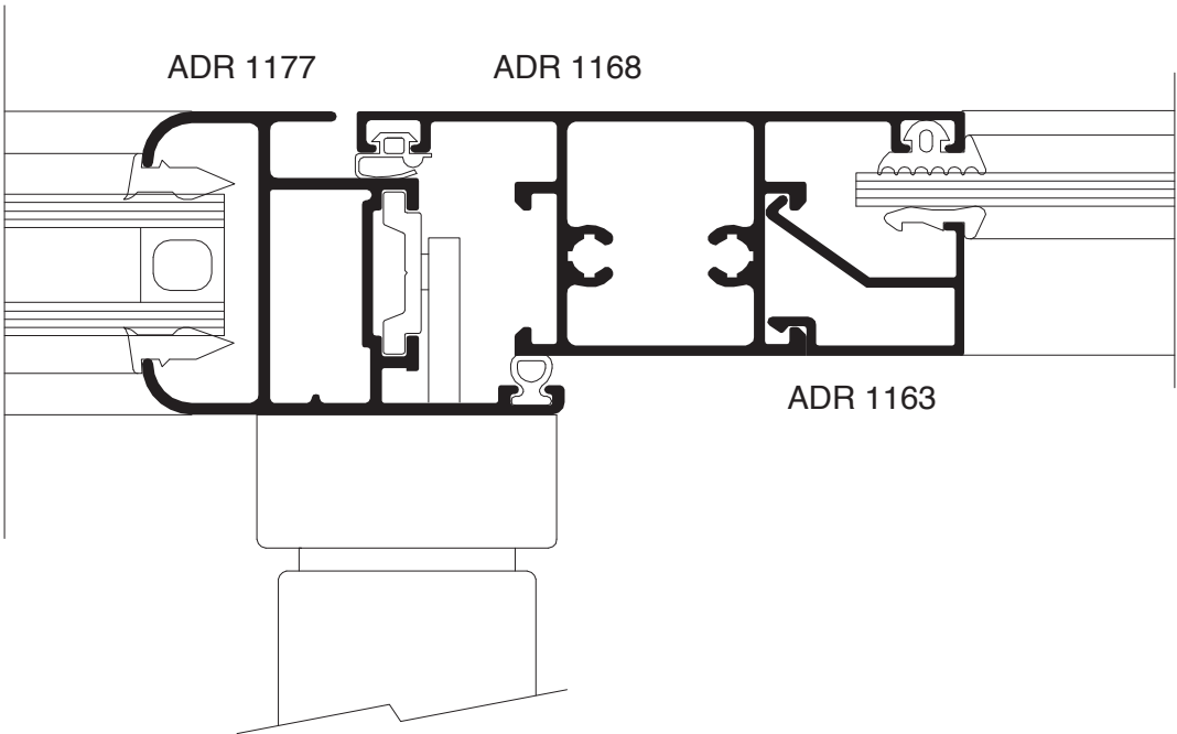
Secciones (Escala 1:1)
