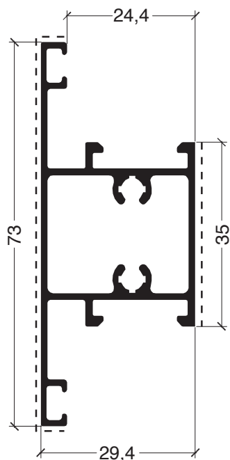
ADR 1168 Travesaño Paño Fijo 0,811 kg/m
