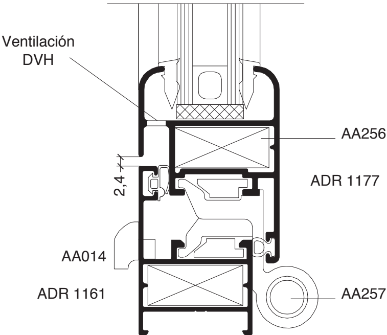
Secciones (Escala 1:1)
