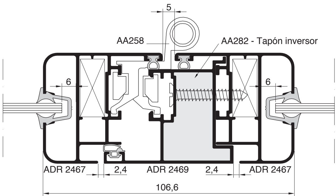
Secciones (Escala 1:1)
