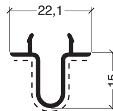
ADR 222 Encuentro central 4 hojas 0,181 kg/m Exclusivo ADR 53A
