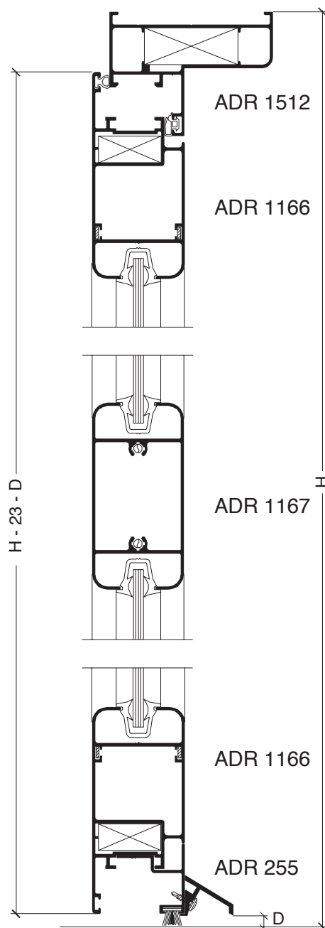
Puerta de una hoja
