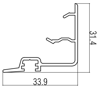
ADR 1516 0.290 KG/M
