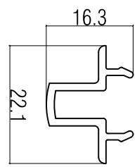
ADR 1651 0.190 KG/M
