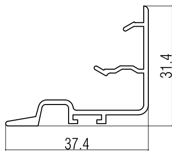
ADR 262 0.309 KG/M
