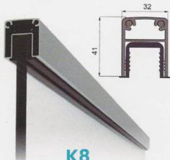
K8 Pasamanos chico
